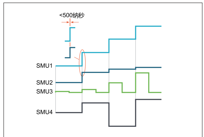
TSP-Link 系统中的所有通道都可同步到 500 ns 以下
