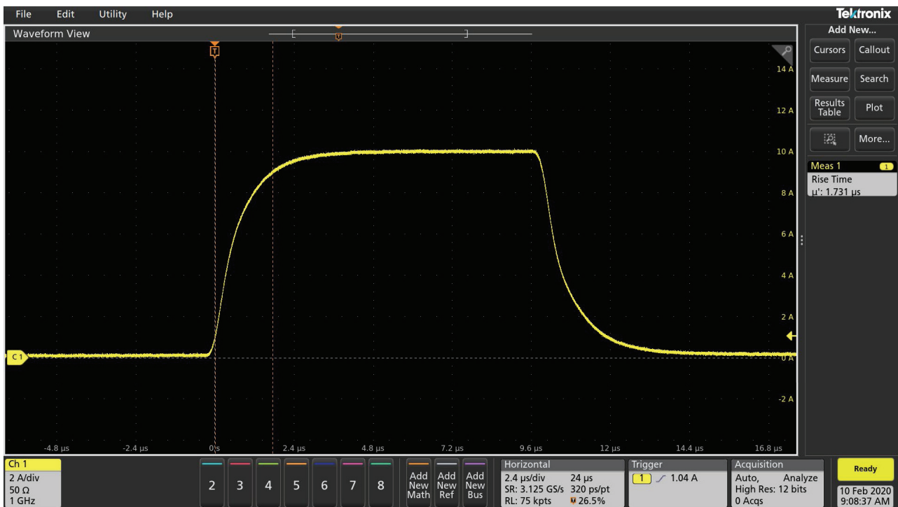
2610B-PUSLE 的脉冲输出性能。
