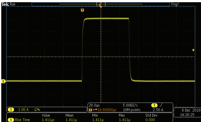
2601B-PULSE 无超调和 1.4 \mu s 上升时间
