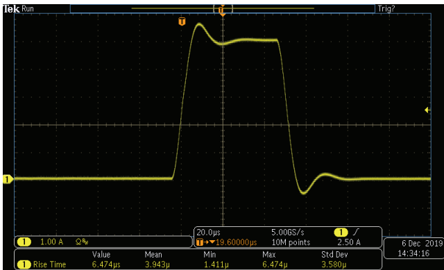
竞争对手 SMU 典型的脉冲输出上升时间 6.47 \mu s
